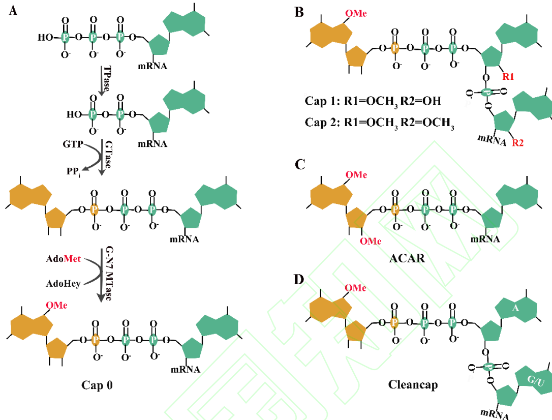
图 3 酶法加帽和帽类似物示意图 [24,35]
